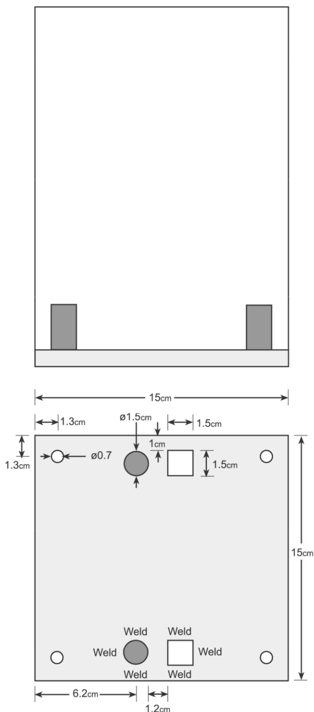
Rysunek podstawy
